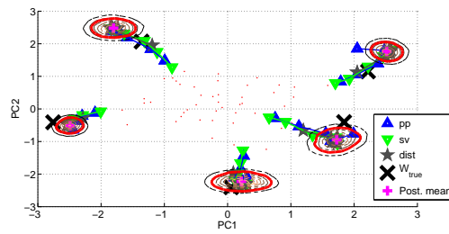
(b) BayesNMF-Vol with posterior mean endmember estimates.
