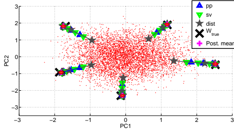
(b) BayesNMF-Vol with posterior mean endmember estimates.
